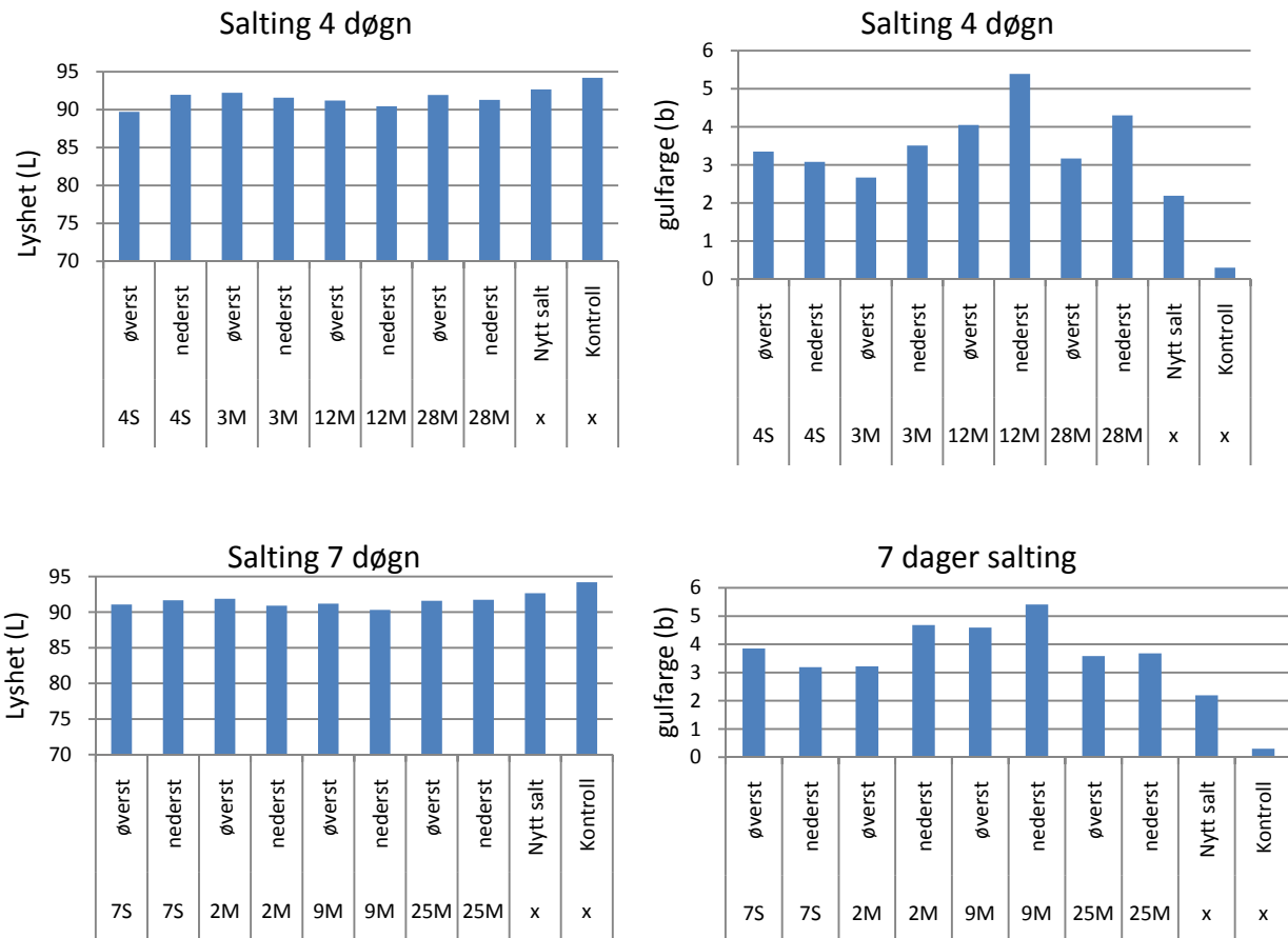
Figur 6.8: Lyshet og gulfarge for prøver fra salt brukt i 4 døgner pickelsalting og nytt salt (2 øverste figurer) og for salt brukt i 7 døgner pickelsalting og nytt salt (2 nederste figurene) (hvit = 100, gul = 60). Øverst og nederst refererer til øverst og nederst i pall. S = saltedøgner, M = modningsdøgner.
